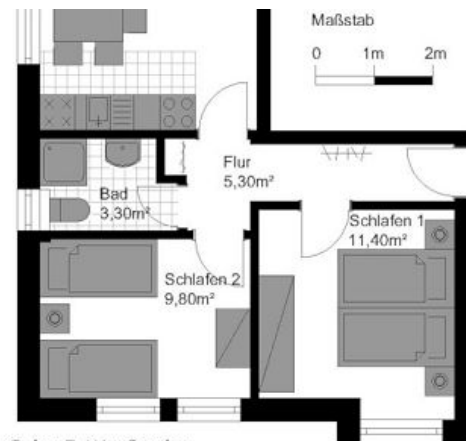
Grundriss B
